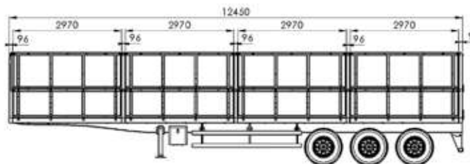
LIBRELATO | CAIXA DE CARGA SEMIRREBOQUE 3 EIXOS 12,50m
