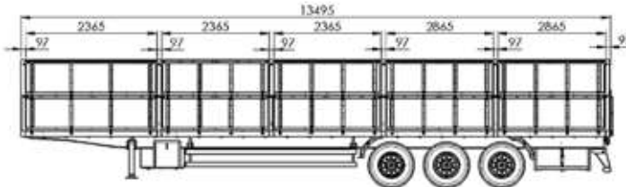
NOMA | CAIXA DE CARGA SEMIRREBOQUE 3 EIXOS 13,50m
