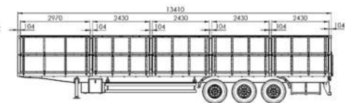
GUERRA | CAIXA DE CARGA SEMIRREBOQUE 3 EIXOS 13,50m
