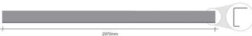
PERFIL LATERAL DA CARRETA SEM FURAÇÃO SP323 - 2970mm - ch. 4,25mm - 25,000kg SP323A - 2230mm - ch. 4,25mm - 18,800kg SP323B - 2590mm - ch. 4,25mm - 21,840kg
