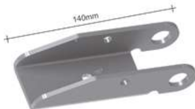
DOBRADIÇA TOMBADOR INFERIOR - 140mm SP428 - ch. 4,25mm - 0,290kg SP428B - SEM PINTURA (10 unidades)
