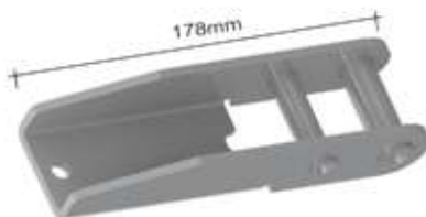
DOBRADIÇA DA TAMPA MODERNA - 178mm SP279 - ch. 4,25mm - 0,540kg SP279B - SEM PINTURA (25 unidades)
