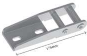
DOBRADIÇA DA TAMP MODERNA - 174mm SP350 - ch. 4,25mm - 0,500kg SP350B - SEM PINTURA (25 unidades)
