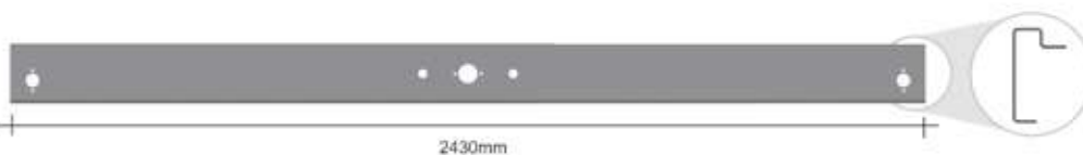
PERFIL DIANTEIRO DA CARRETA - 2430mm SP322 - ch. 4,25mm - 24,000kg
