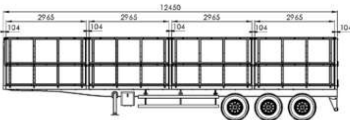
GUERRA | CAIXA DE CARGA SEMIRREBOQUE 3 EIXOS 12,50m
