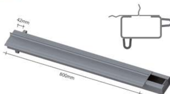
FUEIRO DE CANTO INFERIOR DIREITO/ESQUERDO COM FRISO ECO+
