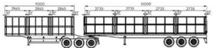
NOMA | CAIXA DE CARGA BITRENÇÃO 9 EIXOS 9,40m + 11,50m
