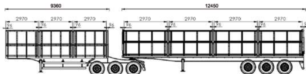
LIBRELATO | CAIXA DE CARGA BITRENÇÃO 9 EIXOS 9,50m + 12,50m
