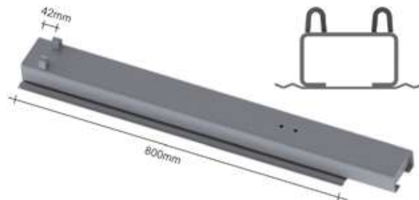
FUEIRO LATERAL INFERIOR COM FRISO ECO+
