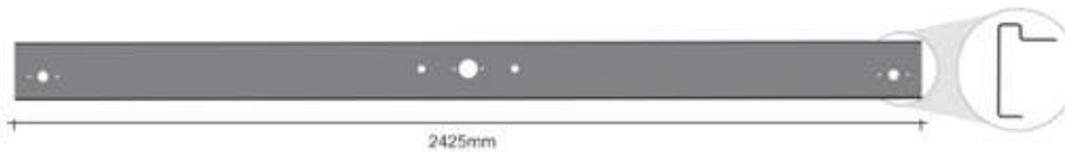
PERFIL DIANTEIRO DA CARRETA BRASILIS/ LINHA R - 2425mm SP219A - ch. 4,25mm - 23,490kg
