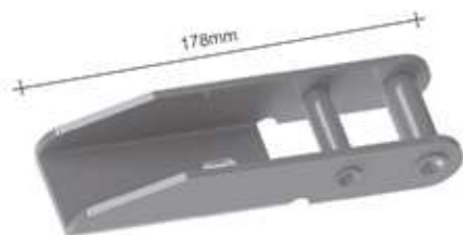
DOBRADIÇA DA TAMPA - 178mm SP427 - ch. 4,25mm - 0,550kg SP427B - SEM PINTURA (25 unidades)
