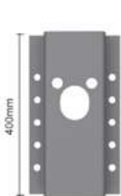
FIXADOR CONJUNTO APARELHO LEVANTAMENTO PÉ MECÂNICO MODERNO 400mm SP367 - ch. 6,35mm - 5,700kg
