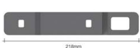
ENGATE FÊMEA DA TAMPA SUPERIOR - 218mm SP044 - ch. 6,35mm - 0,370kg * SEM PINTURA (25 unidades)
