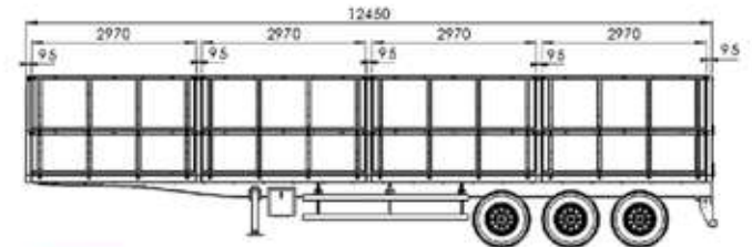
RANDON | CAIXA DE CARGA SEMIRREBOQUE 3 EIXOS 12,50m
