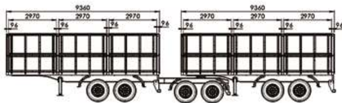
LIBRELATO | CAIXA DE CARGA RODOTREM 9 EIXOS 9,40m
