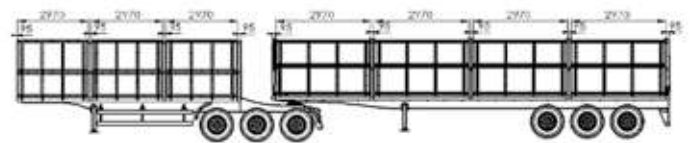
RANDON | CAIXA DE CARGA BITRENÇÃO 9 EIXOS 9,40m + 12,50m
