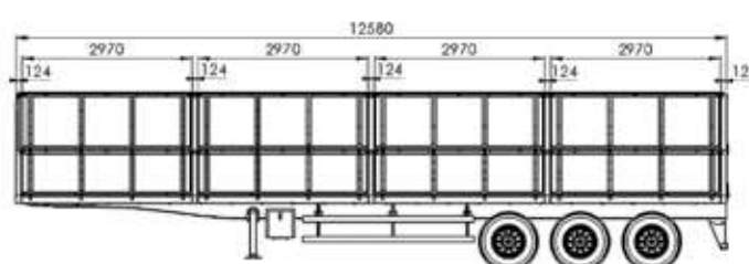
FACCHINI | CAIXA DE CARGA SEMIRREBOQUE 3 EIXOS 12,50m
