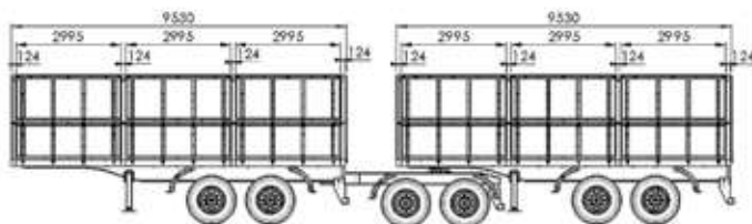
FACCHINI | CAIXA DE CARGA RODOTREM 9 EIXOS 9,50m
