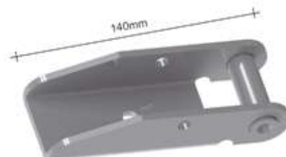
DOBRADIÇA TOMBADOR SUPERIOR - 140mm SP428A - ch. 4,25mm - 0,320kg SP428AB - SEM PINTURA (10 unidades)
