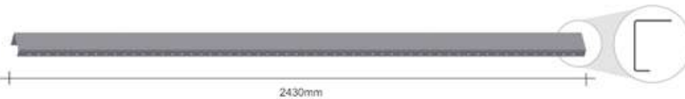
PERFIL TRASEIRO LINHA ECO+ - 2430mm SP795 - ch. 4,25mm - 24,620kg
