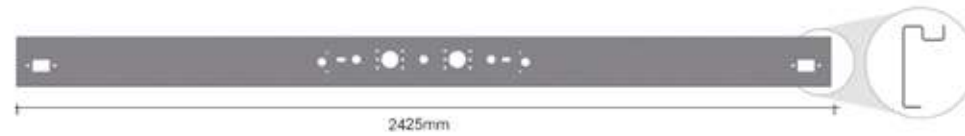
PERFIL DIANTEIRO DA CARRETA NEW R FREIOS ABS ASSOALHO DE FERRO - 2425mm SP219C - ch. 4,25mm - 23,320kg
