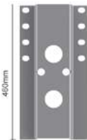
FIXADOR CONJUNTO APARELHO LEVANTAMENTO PÉ MECÂNICO 460mm SP496 - ch. 6,35mm - 7,000kg
