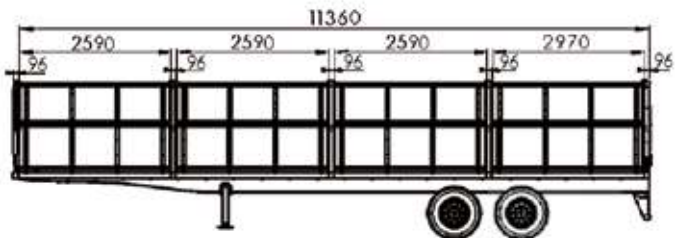
LIBRELATO | CAIXA DE CARGA SEMIRREBOQUE 2 EIXOS 11,50m
