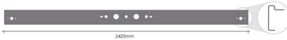
PERFIL DIANTEIRO DA CARRETA LINHA R ASSOALHO MADEIRA - 2425mm SP219B - ch. 4,25mm - 23,340kg
