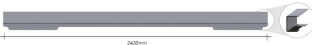
PERFIL TRASEIRO DA CARRETA - 2430mm SP324 - ch. 4,25mm - 24,000kg
