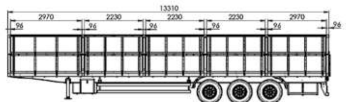
LIBRELATO | CAIXA DE CARGA SEMIRREBOQUE 3 EIXOS 13,50m
