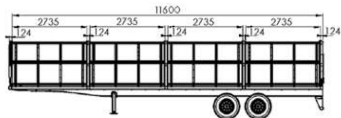
FACCHINI | CAIXA DE CARGA SEMIRREBOQUE 2 EIXOS 11,60m
