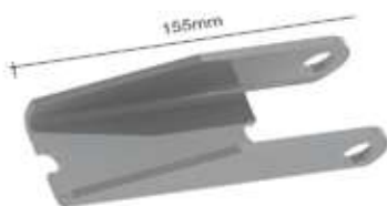
DOBRADIÇA DO TOMBADOR INFERIOR - 155mm SP047 - ch. 4,25mm - 0,400kg SP047B - SEM PINTURA (10 unidades)
