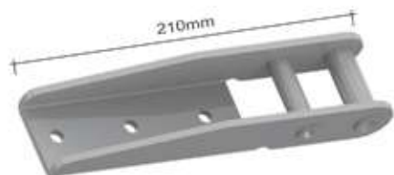
DOBRADIÇA DA TAMPA ANTIGA - 210mm SP046 - ch. 4,25mm - 0,630kg SP046B - SEM PINTURA (25 unidades)
